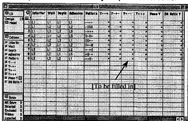
Fig. 2a: Taguchi Design
