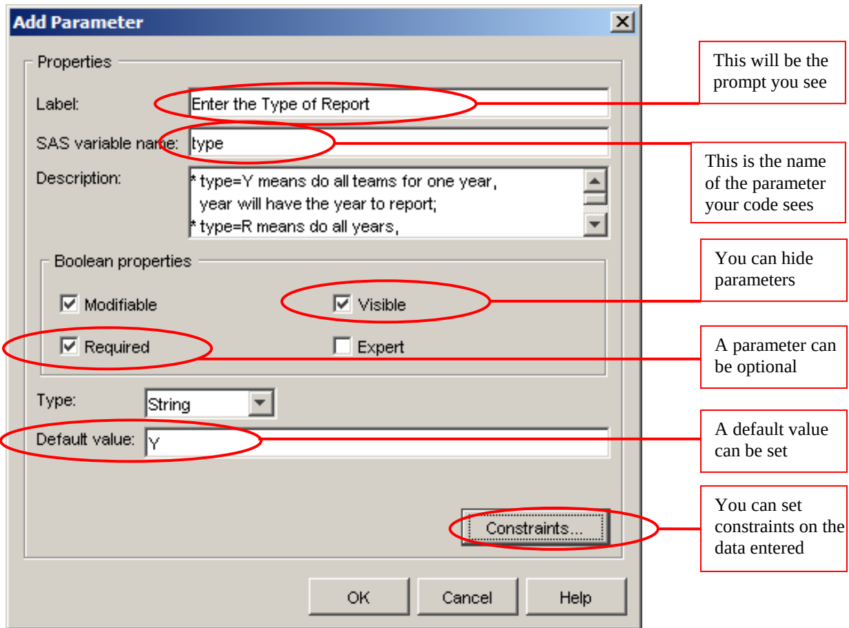
FIGURE 5: PARAMETER VALUES
